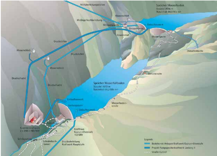
Darstellung des Pumpspeicherkraftwerkes Limberg II
